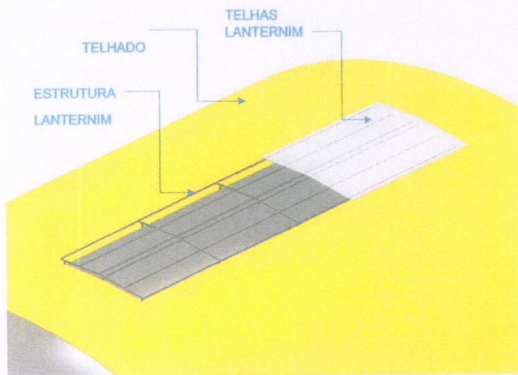
Fig. 04 – Lanterna
