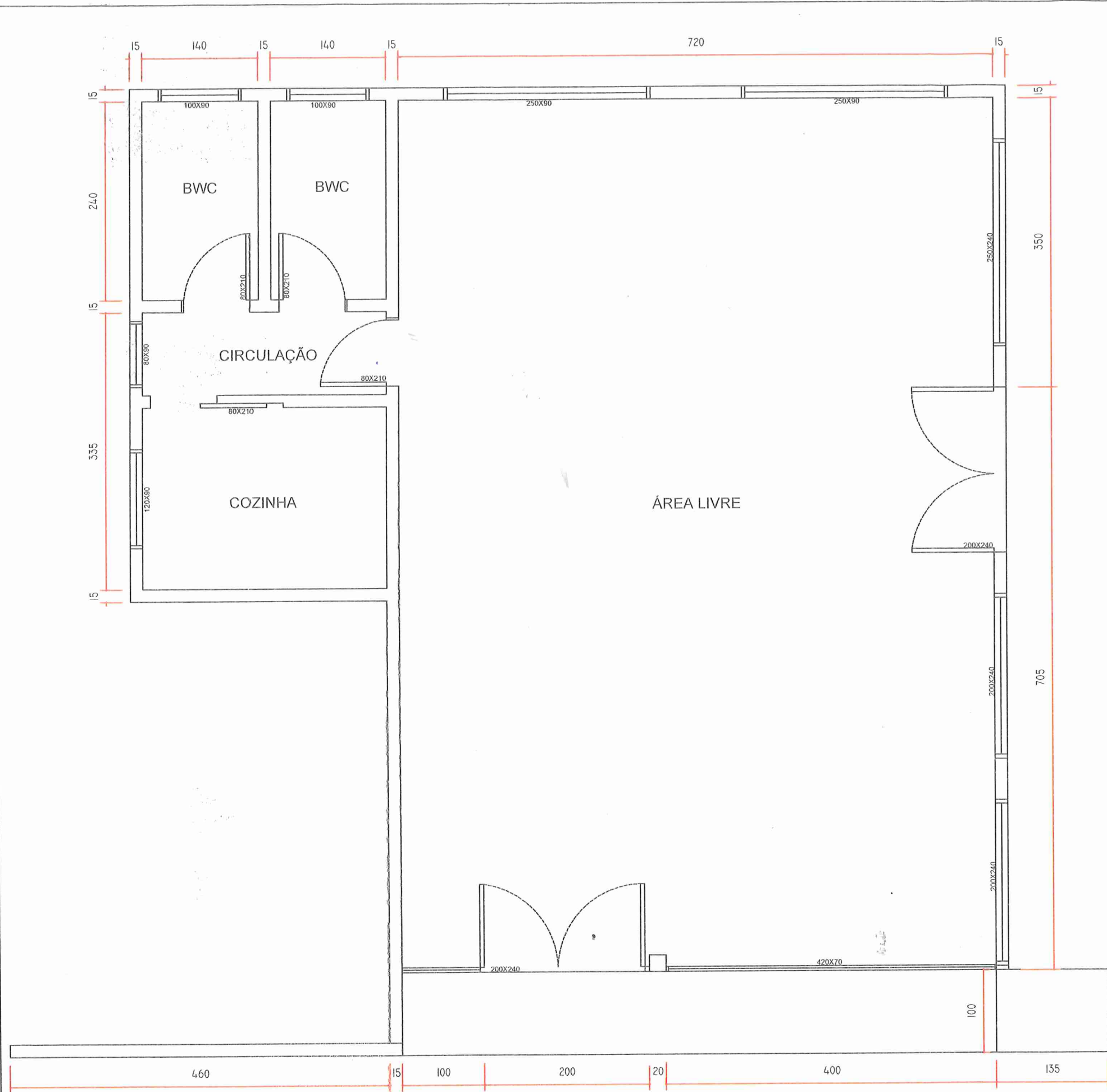
Planta baixa- Capéla Mortuária Área:103,07m²
